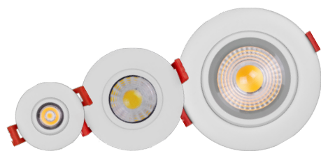
DGDv1
